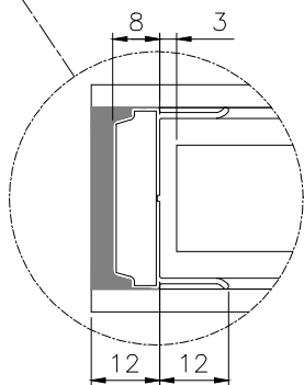
Canalina con guida 32 mm
