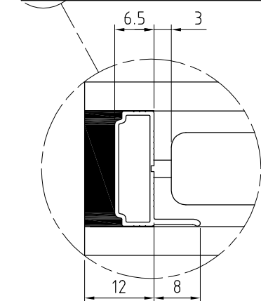
CANALINA RIBASSATA CON ALETTA
