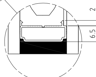
CANALINA RIBASSATA CON INCASTRO
