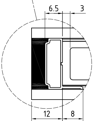
CANALINA RIBASSATA CON ALETTA 20 MM
