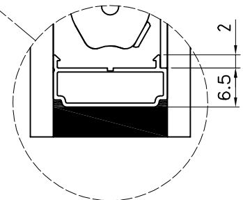
CANALINA RIBASSATA CON INCASTRO 20 MM
