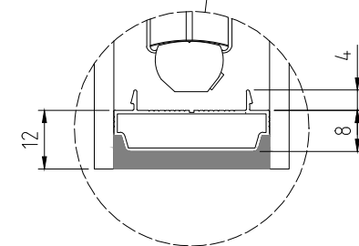
CANALINA ESTRUSA CON INCASTRO
