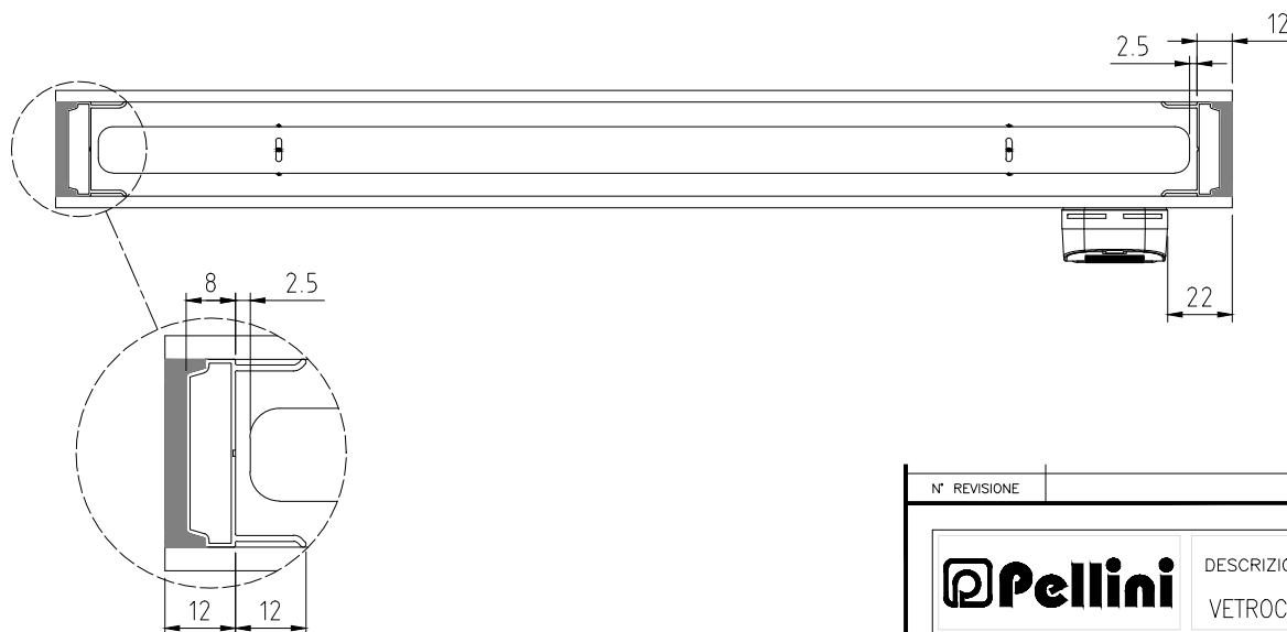
CANALINA ESTRUSA CON GUIDA
