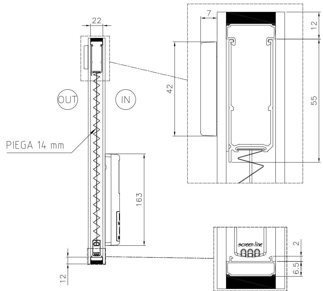
CANALINA ESTRUSA RIBASSATA CON INCASTRO
